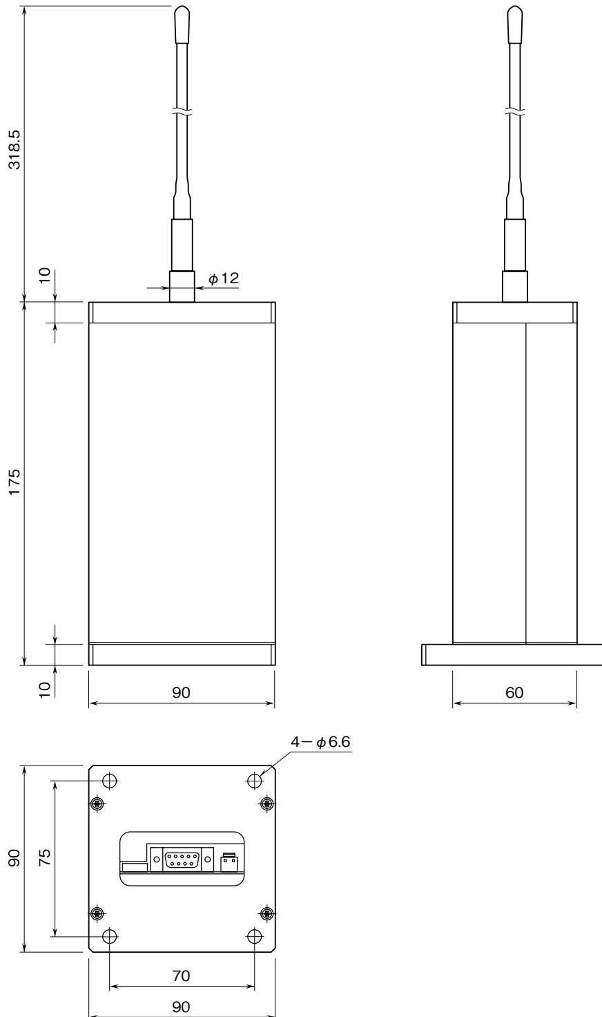
外形寸法図 (単位: mm)
