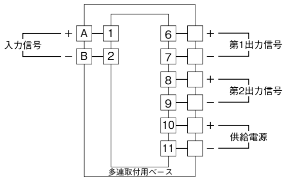
端子接続図
