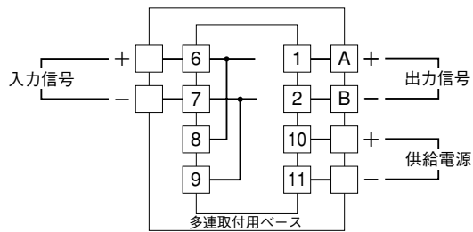
端子接続図
