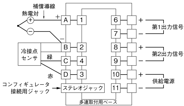
端子接続図
