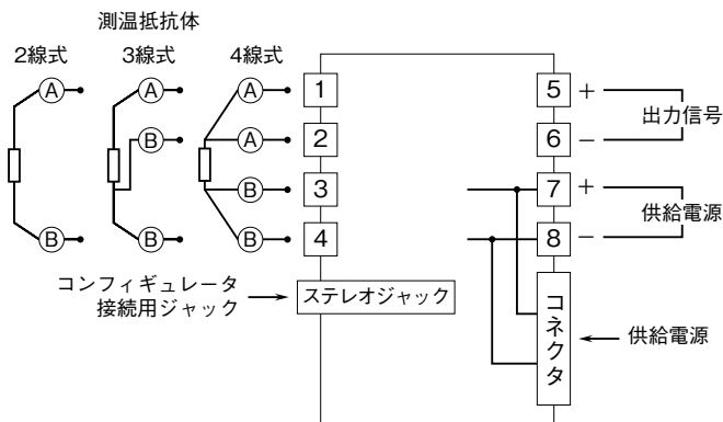
端子接続図
