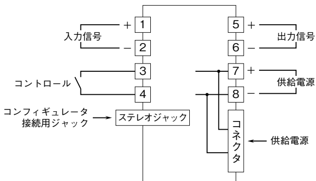
端子接続図
