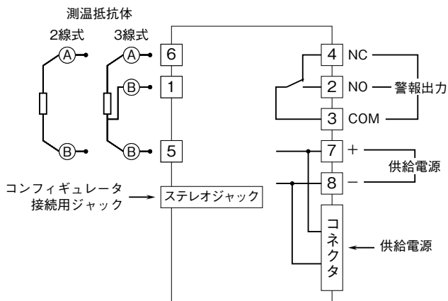
端子接続図
