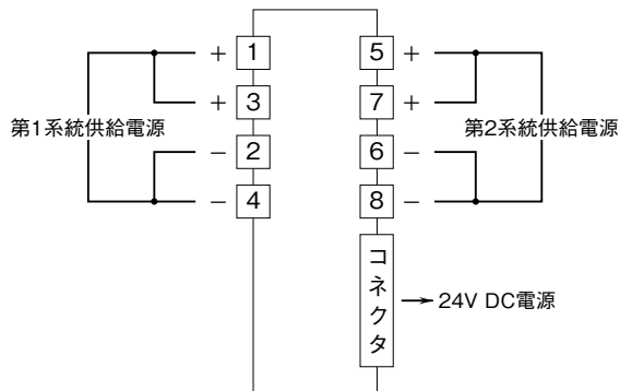
端子接続図
