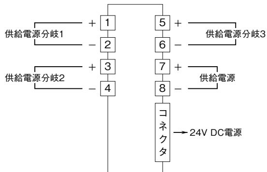
端子接続図
