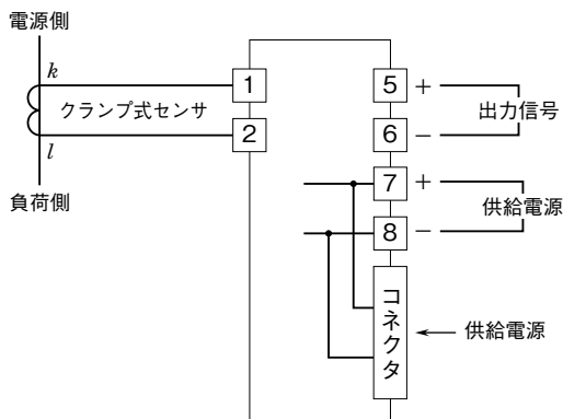
端子接続図
