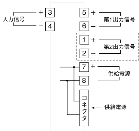
端子接続図
