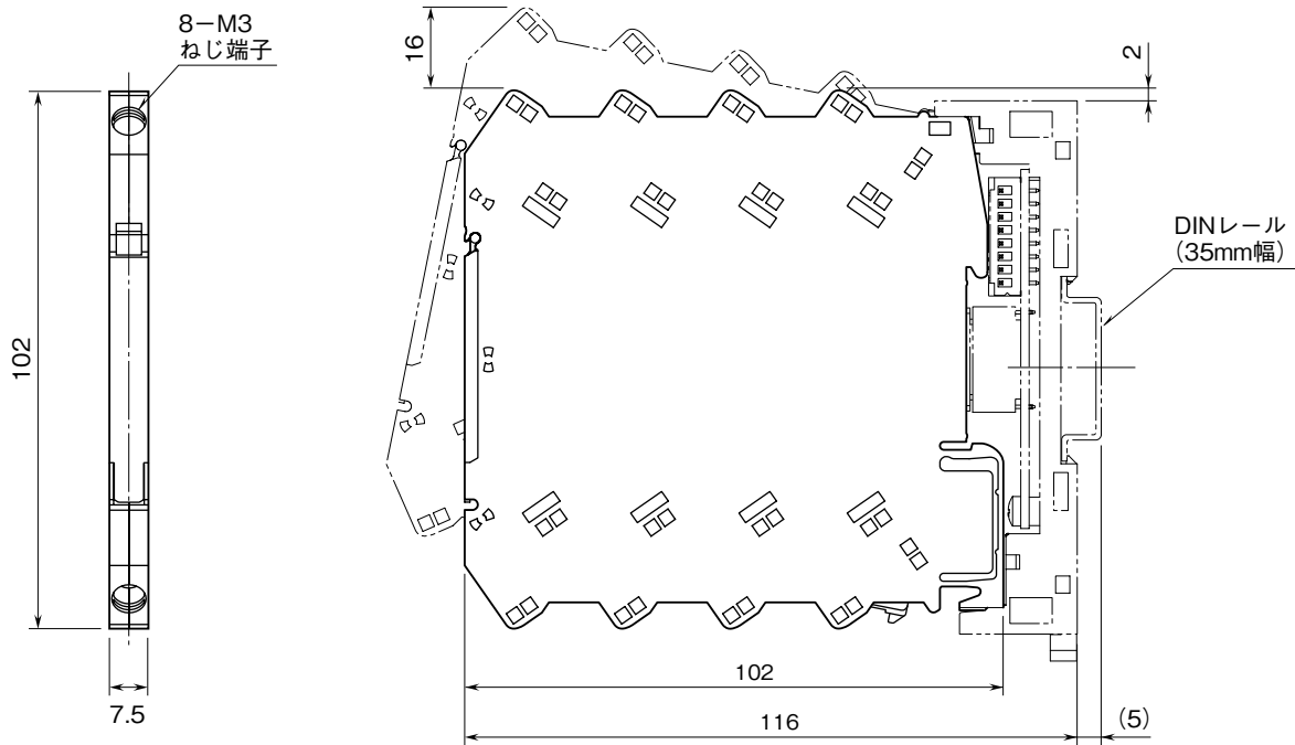
外形寸法図 (単位: mm)
