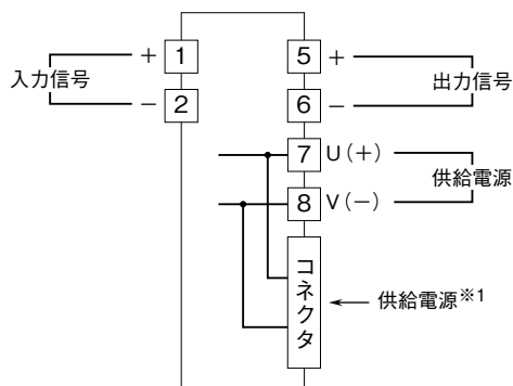
端子接続図
