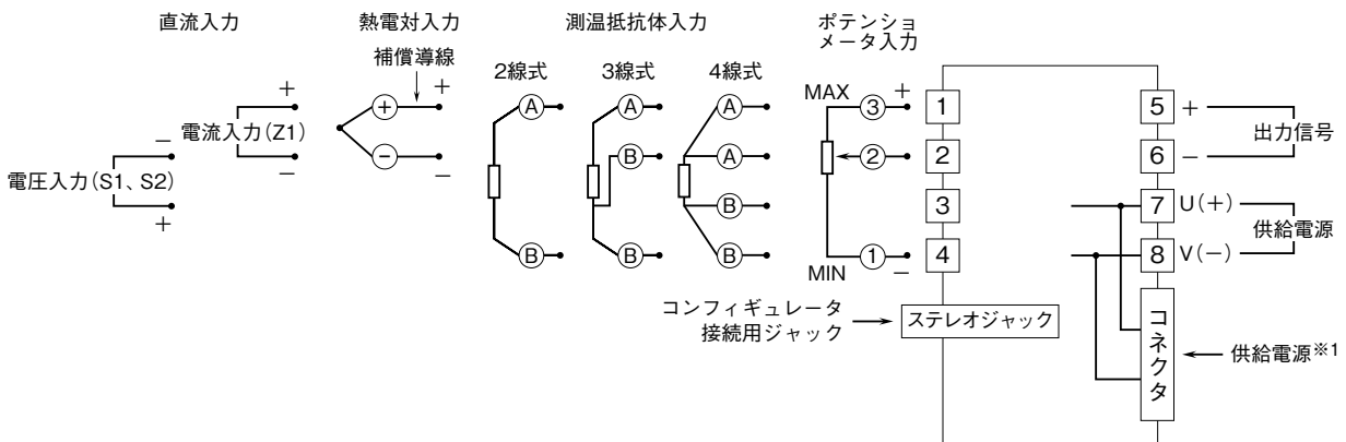
端子接続図
