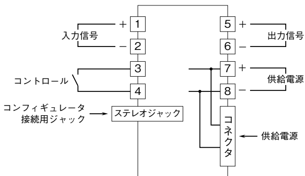
端子接続図
