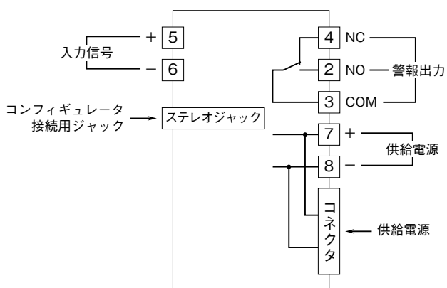
端子接続図
