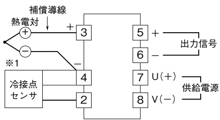
端子接続図
