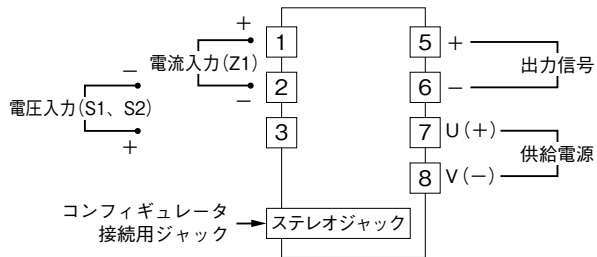
端子接続図
