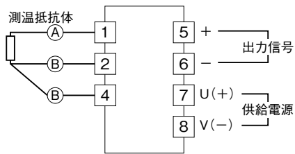
端子接続図
