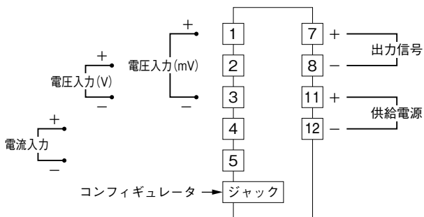
端子接続図
