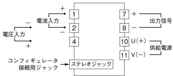
端子接続図
