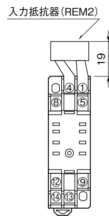
端子番号図 (単位: mm)
