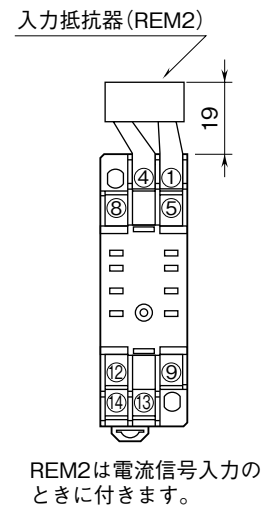
端子番号図 (単位: mm)
