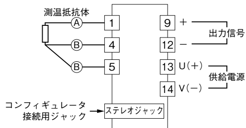
端子接続図
