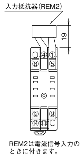
取付寸法図 (単位: mm)
