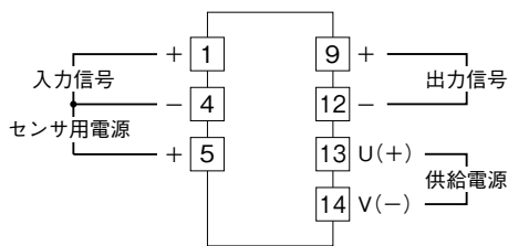
端子接続図
