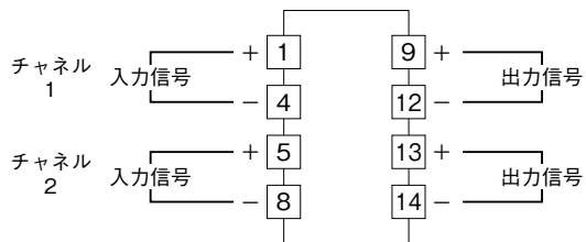
端子接続図
