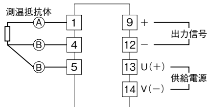
端子接続図
