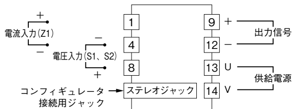
端子接続図
