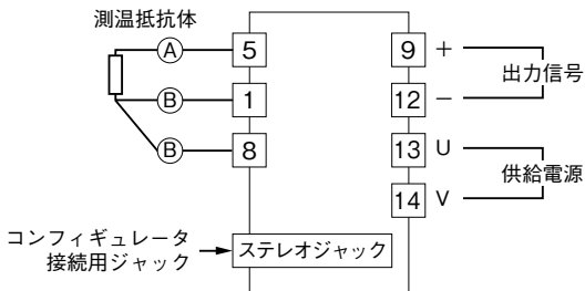
端子接続図
