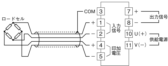
端子接続図
