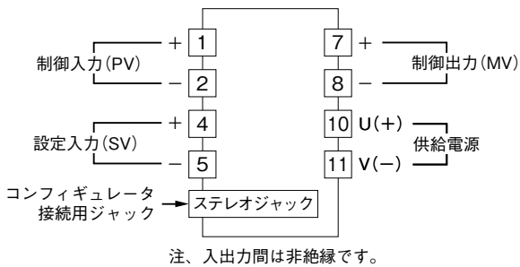
端子接続図
