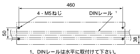
取付寸法図 (単位: mm)
