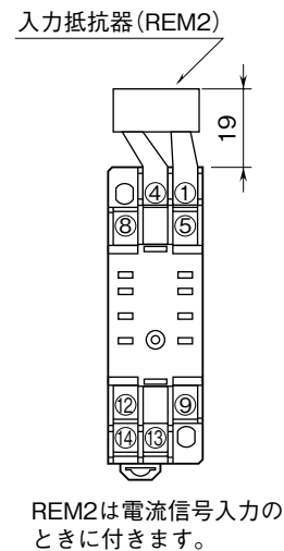
端子番号図 (単位: mm)
