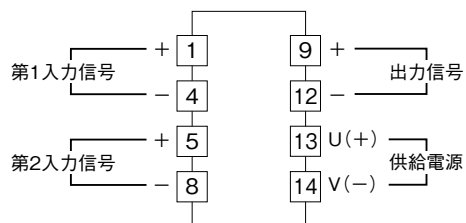
端子接続図
