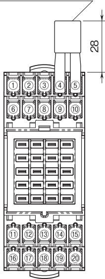
抵抗モジュール (REM3)
