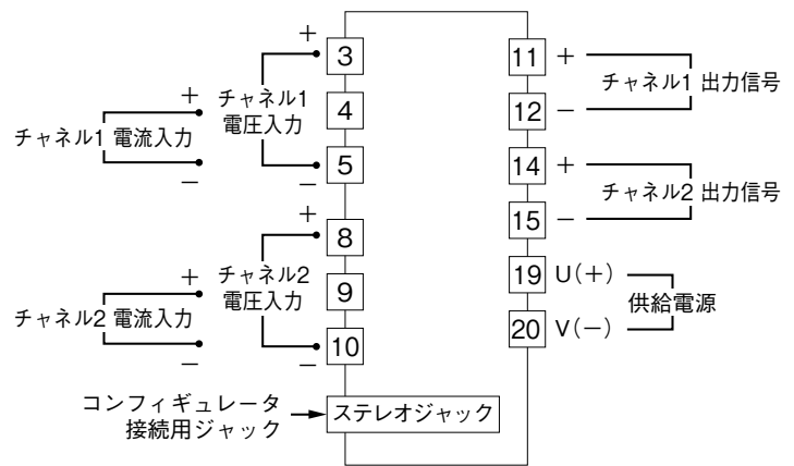
端子接続図
