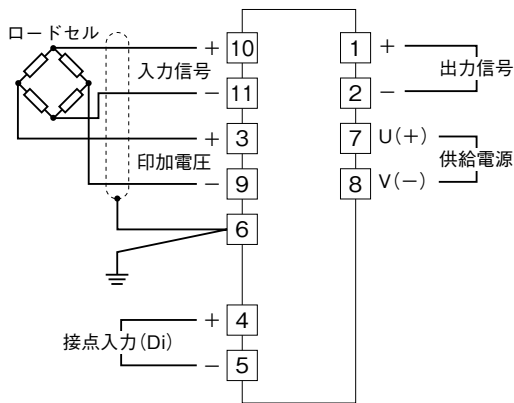
端子接続図
