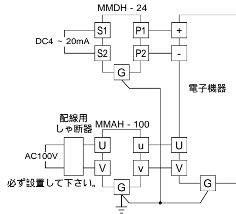
端子接続図
