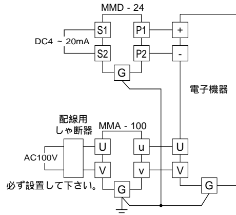
端子接続図
