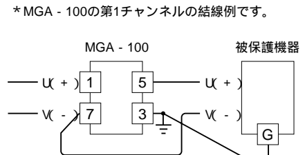
端子接続図
