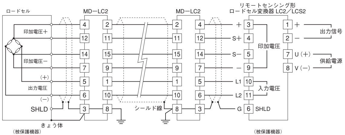
端子接続図
