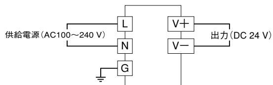
端子接続図
