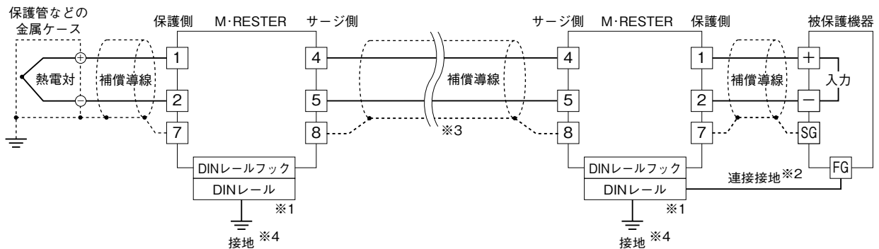
結線要領図
