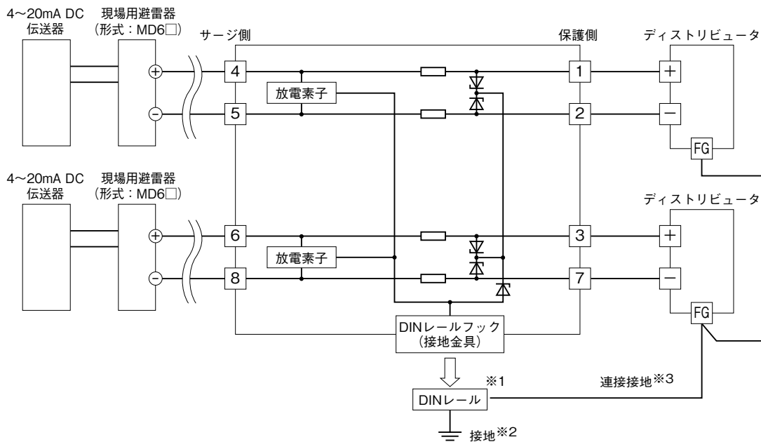
結線要領図
