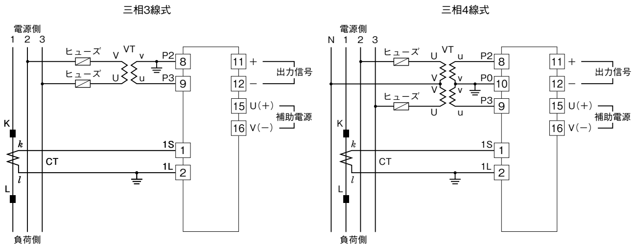
端子接続図
