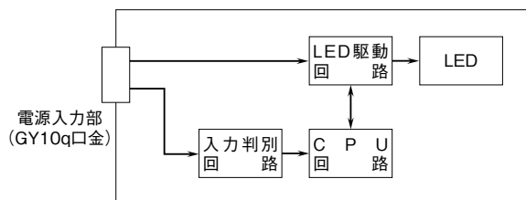
ブロック図
