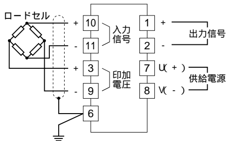
端子接続図
