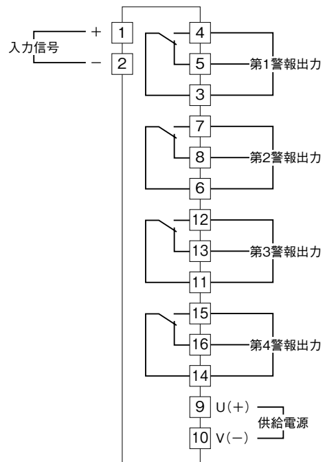
端子接続図
