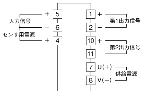
端子接続図
